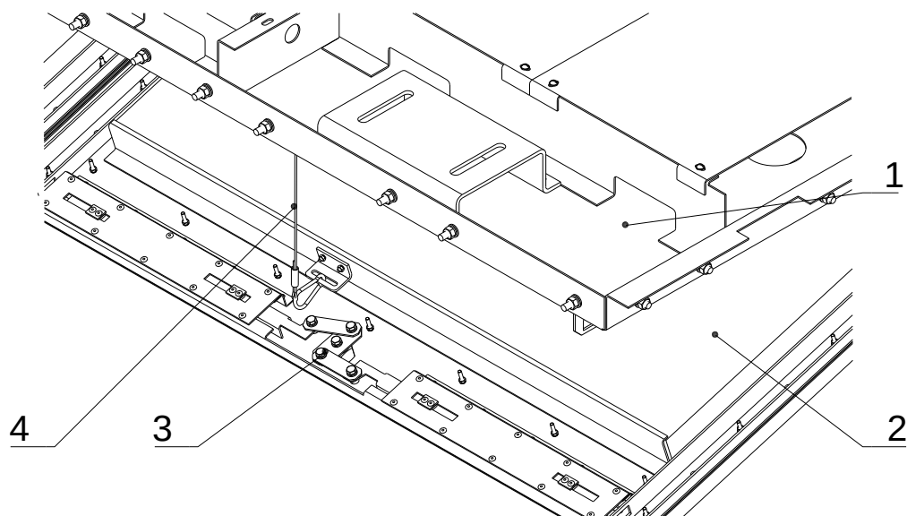
Рис. 59. Установка страховочного каната
