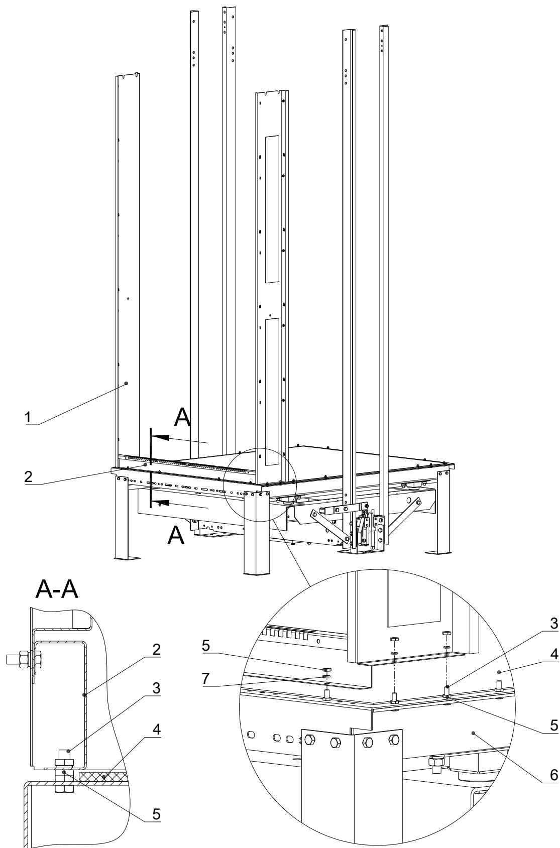
1 – стояк купе, 2 – плинтус, 3 – болт, 4 – покрытие пола, 5 – гайка, 6 – пол, 7 – шайба. Рис. 11.
