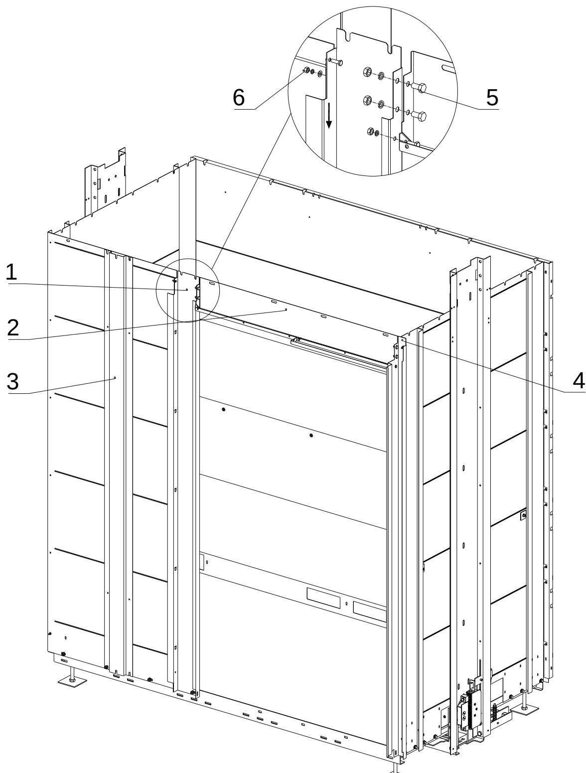
1, 4 – стояк купе, 2 – притолока, 3 – ребро жесткости, 5, 6 – крепёж.
