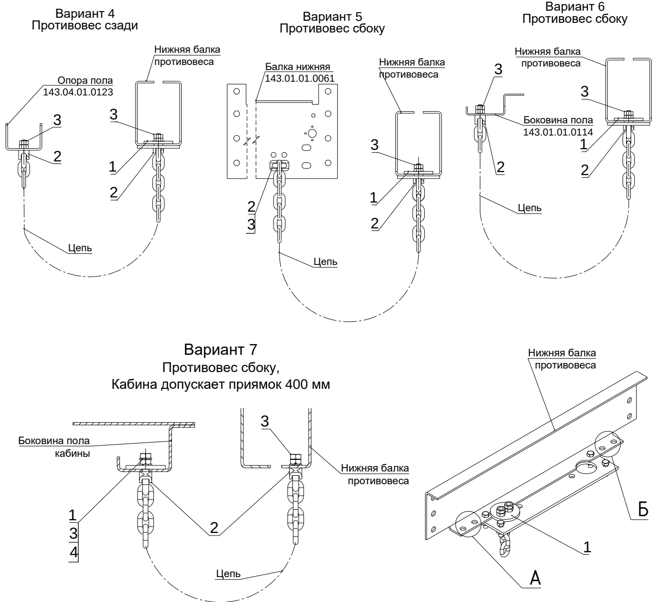
Рис. 73. Монтаж компенсирующей цепи.
