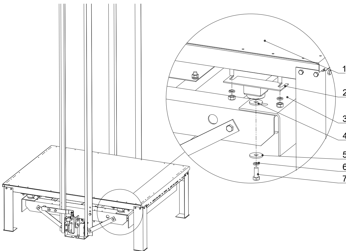
1 – пол, 2 – датчик системы грузовзвешивания, 3 – балка нижняя, 4, 5, - шайба, 6 – гровер, 7 – болт.
