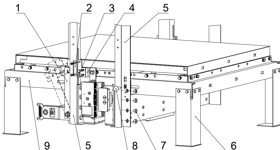
1 – рычаг синхронизатора, 2 – уголок трения, 3, 7, 8 – крепеж, 4 – кронштейн, 5 – стояк, 6 – стойка, 9 – пол в сборе с балкой нижней.
