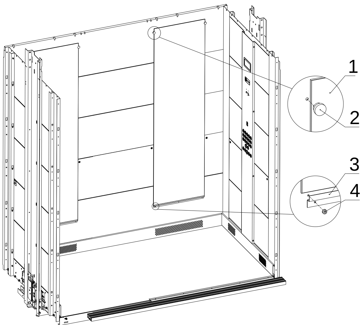
1 – зеркало, 2 – держатель, 3 – планка, 4 - заклепка.
