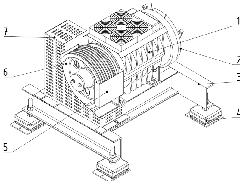
Рис. 63а. Лебёдка безредукторная
